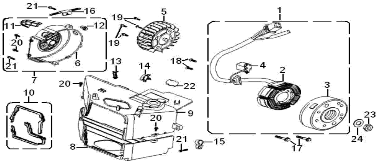
FIG 8 - FAN & ALTERNATOR
